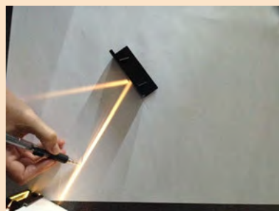
Merk die invalstraal.
