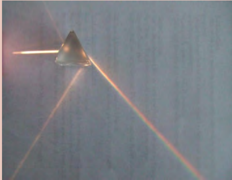
'n Foto van die prisma.
