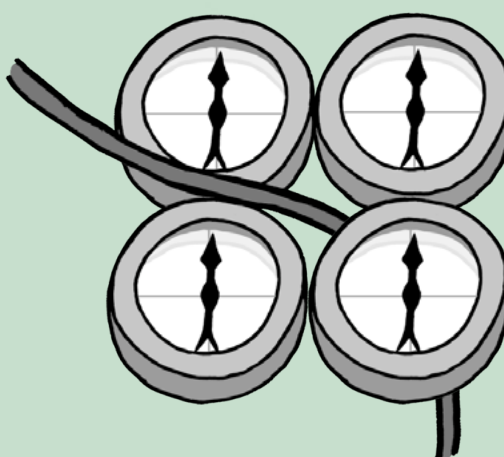
Kompasse wat rondom 'n geleidingsdraad geplaas is.
