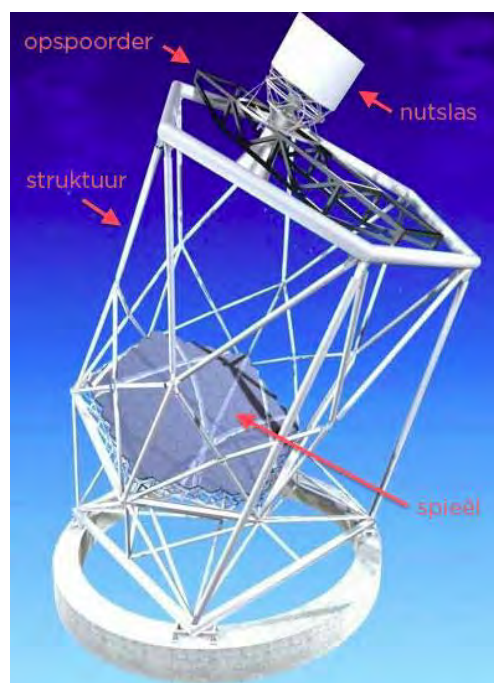
Die struktuur van SALT. (Bron: SALT)
